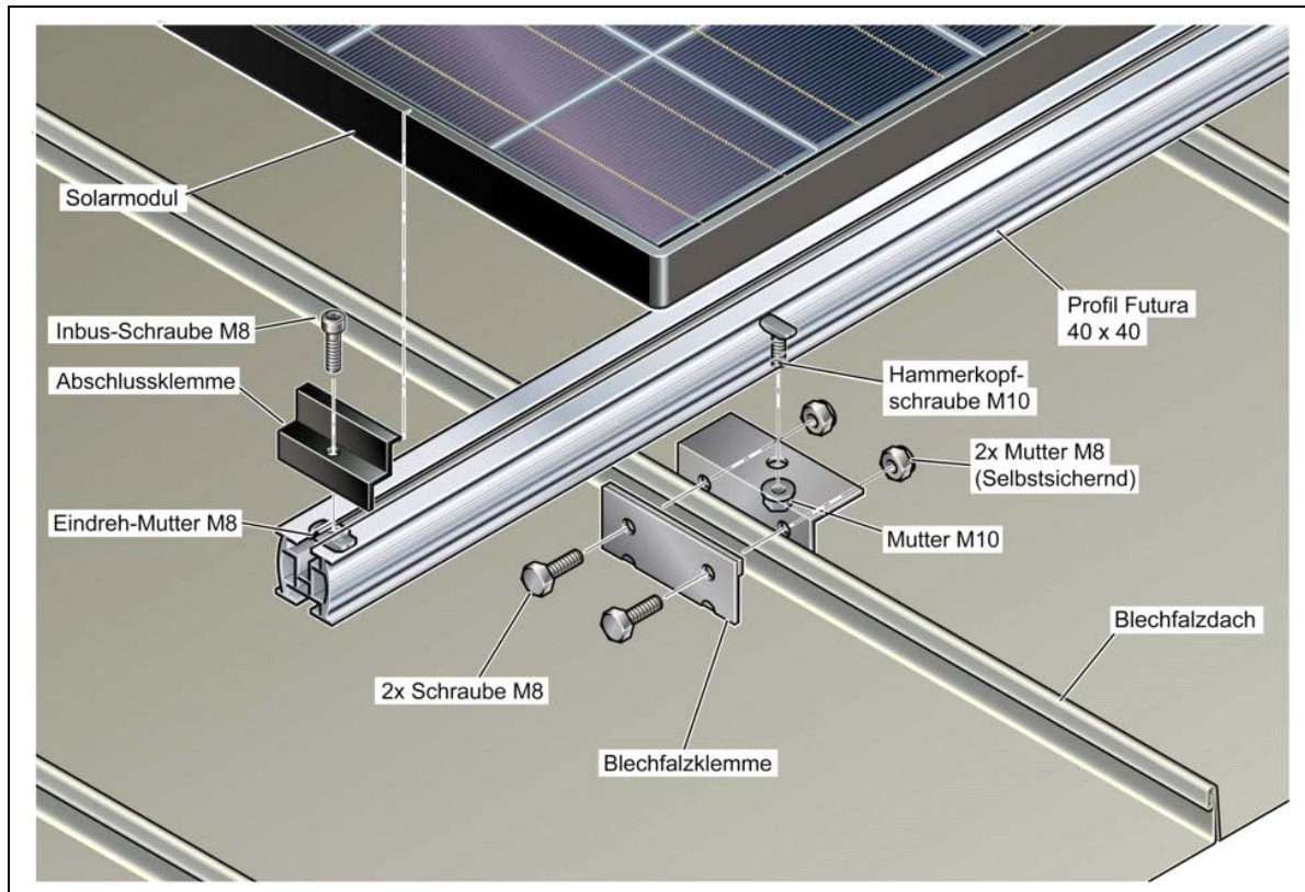
C – Schrägdach Detail Blechfalzklemme - Explosionsdarstellung
