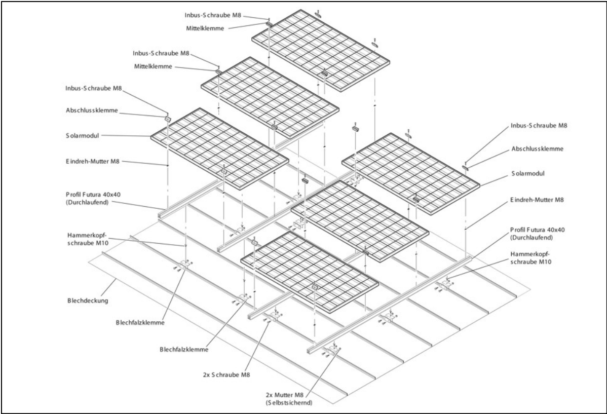
A - Module auf Blechfalzdach - Explosionsdarstellung
