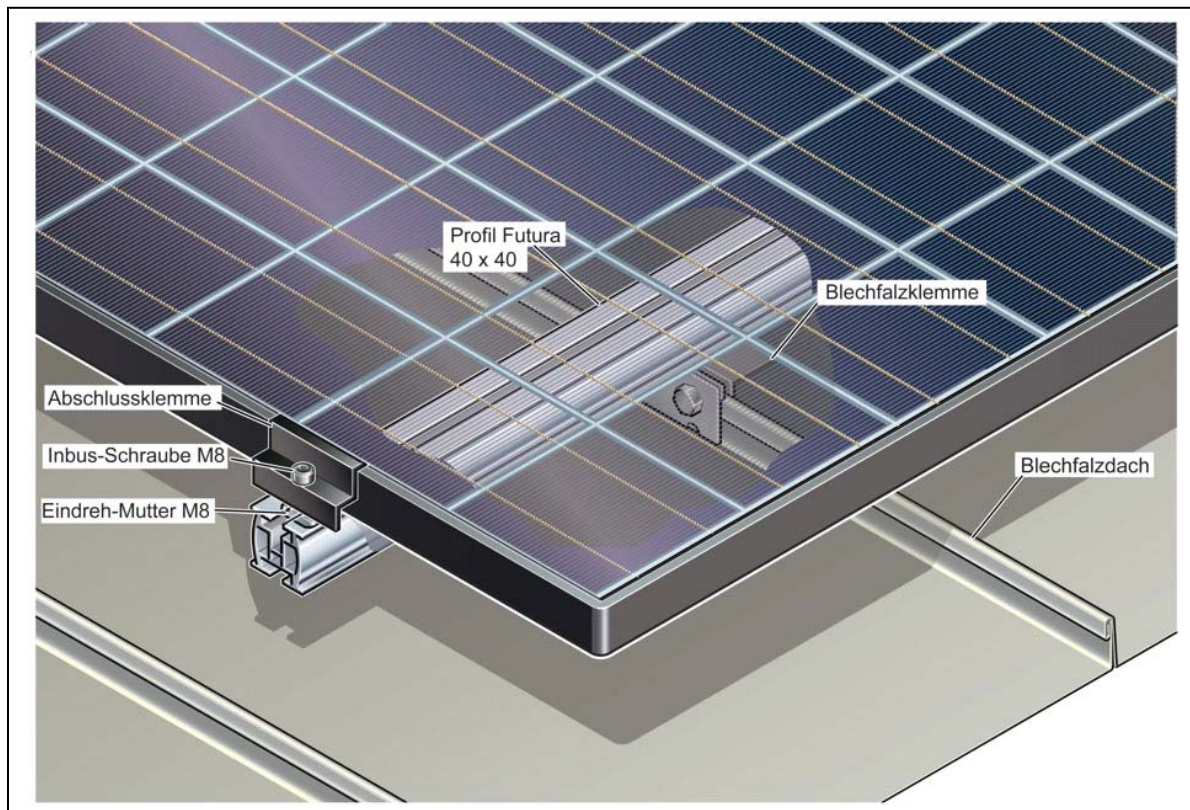
D – Schrägdach Ausschnitt Blechfalzklemme - Zusammenbau
