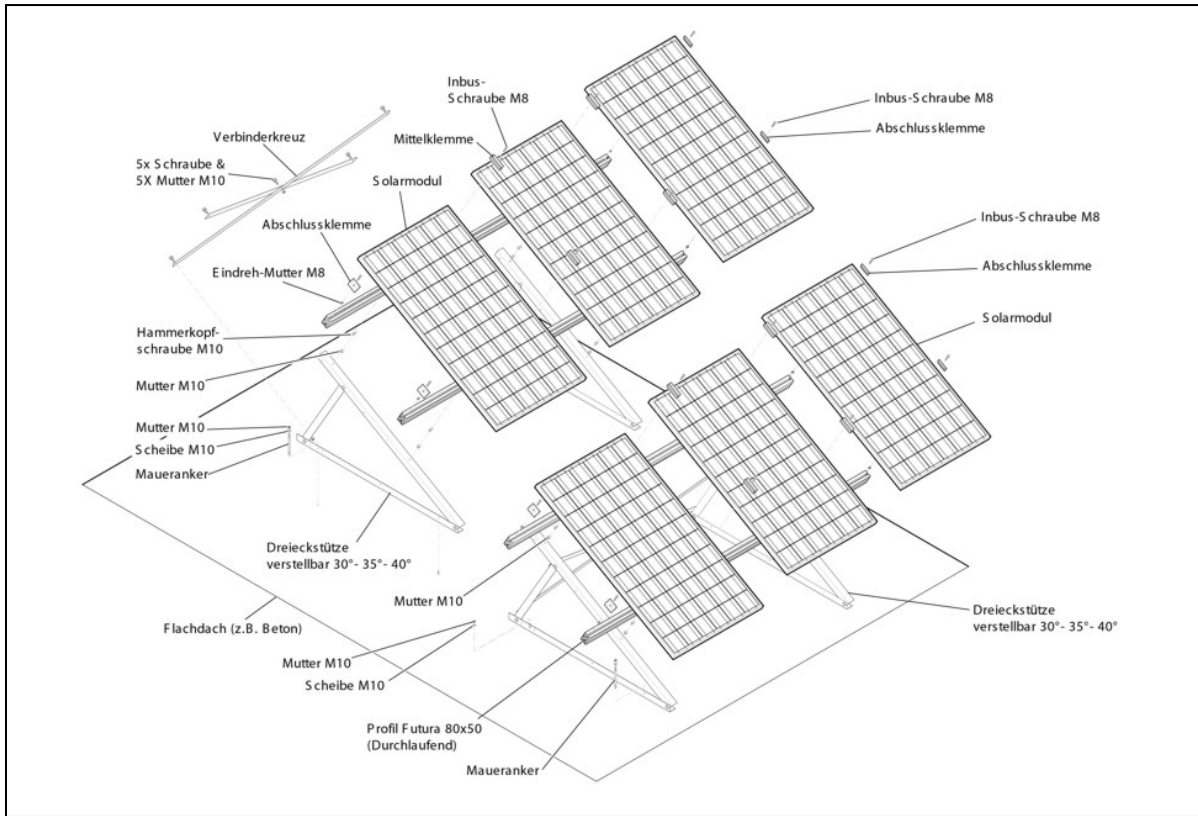
A - Modul auf Flachdach - Explosionsdarstellung
