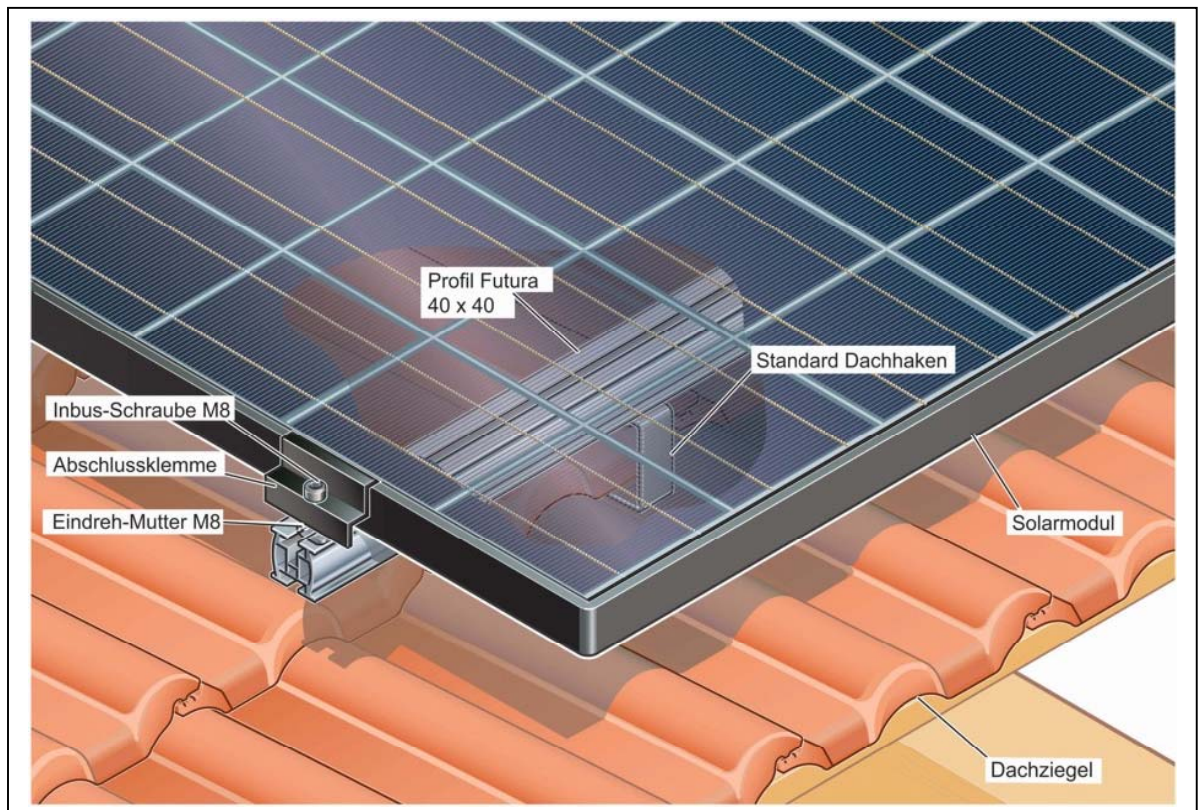
D – Schrägdach Ausschnitt Dachhaken - Zusammenbau
