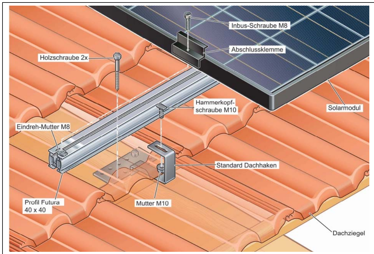
C – Schrägdach Detail Dachhaken - Explosionsdarstellung
