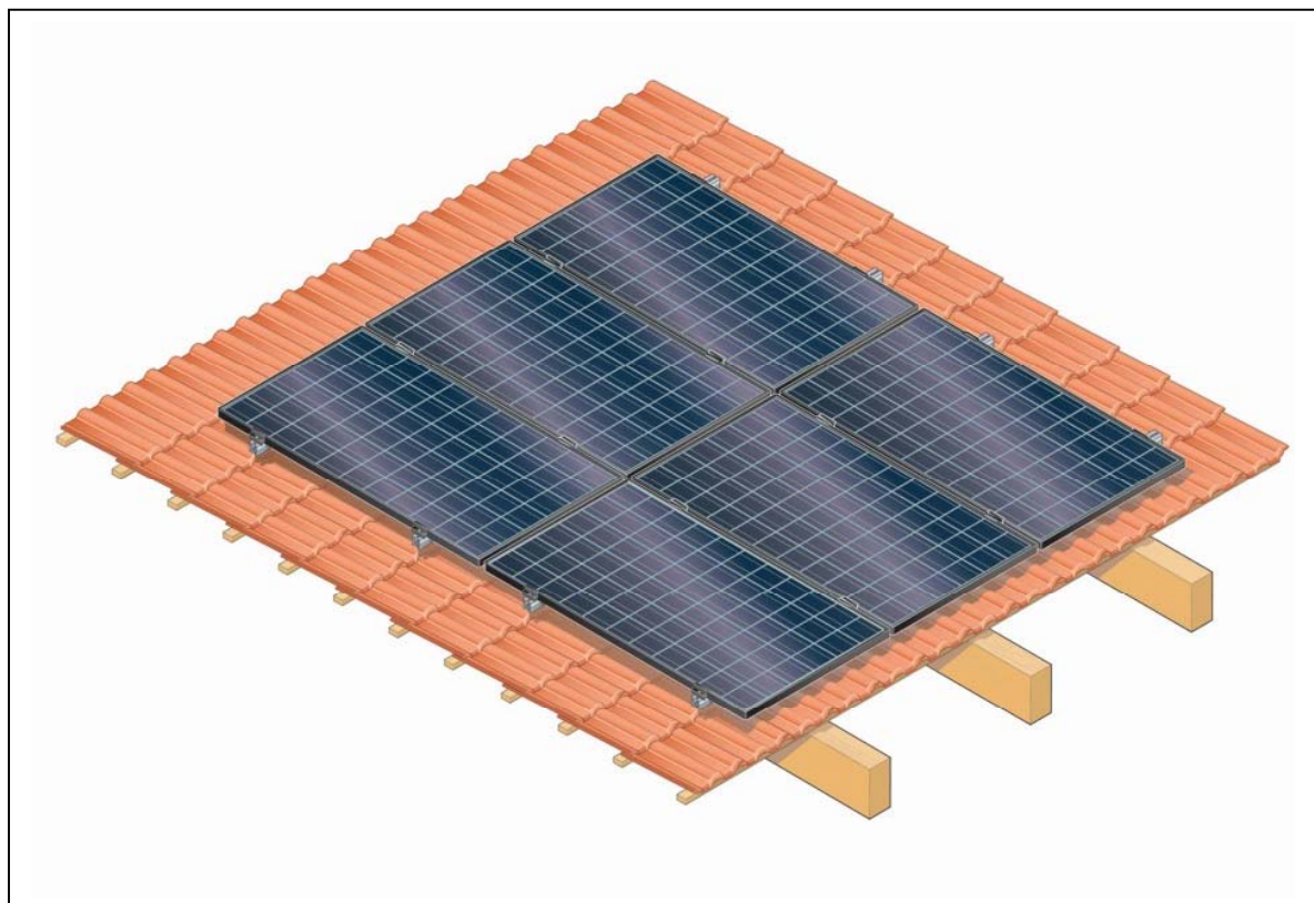
B - Module auf Schrägdach (Ziegeldeckung) - Zusammenbau
