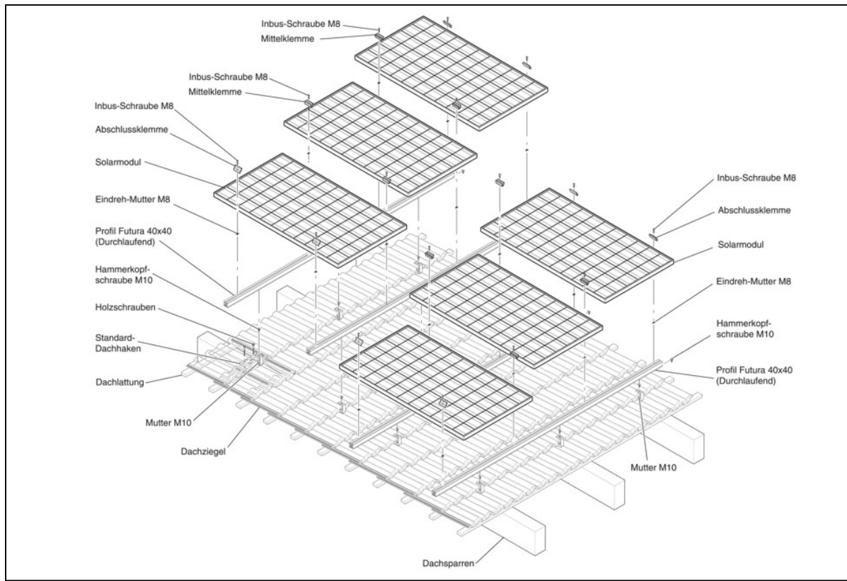
A - Modul auf Schrägdach (Ziegeldeckung) - Explosionsdarstellung
