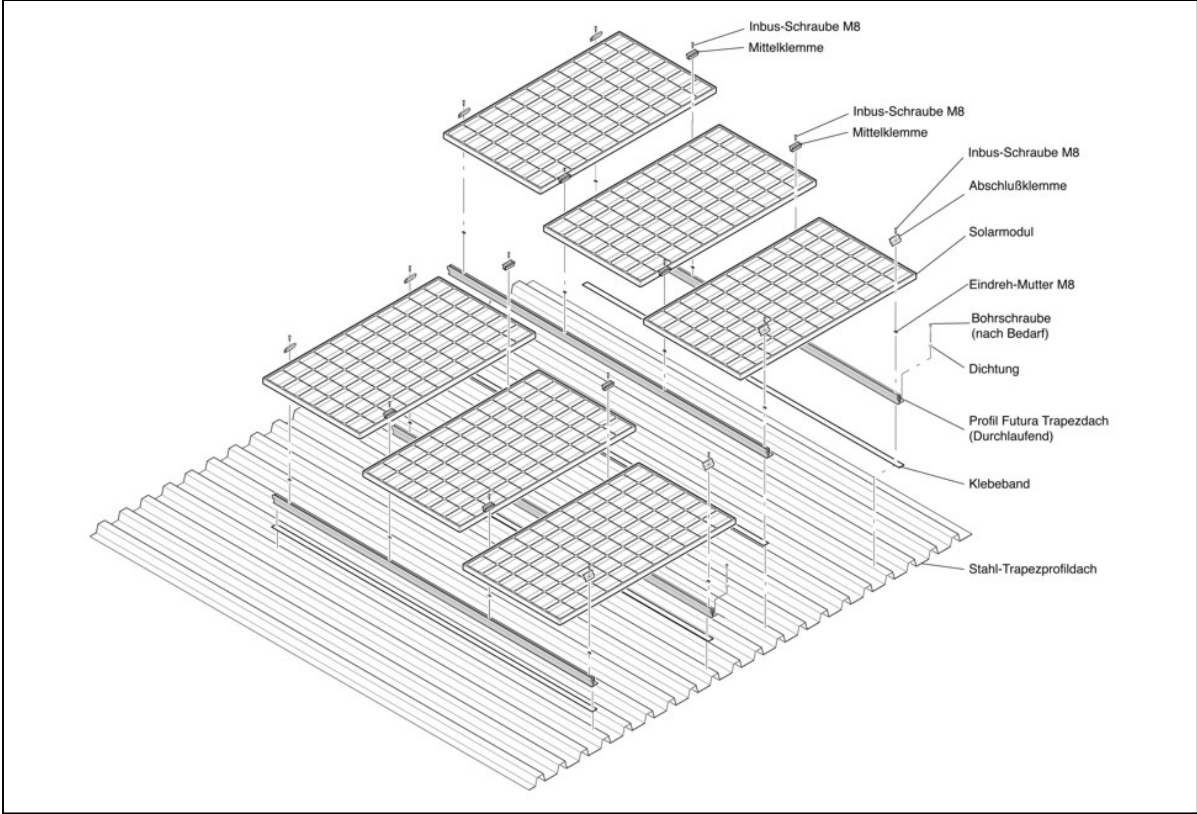
A - Modul auf Trapezdach - Explosionsdarstellung
