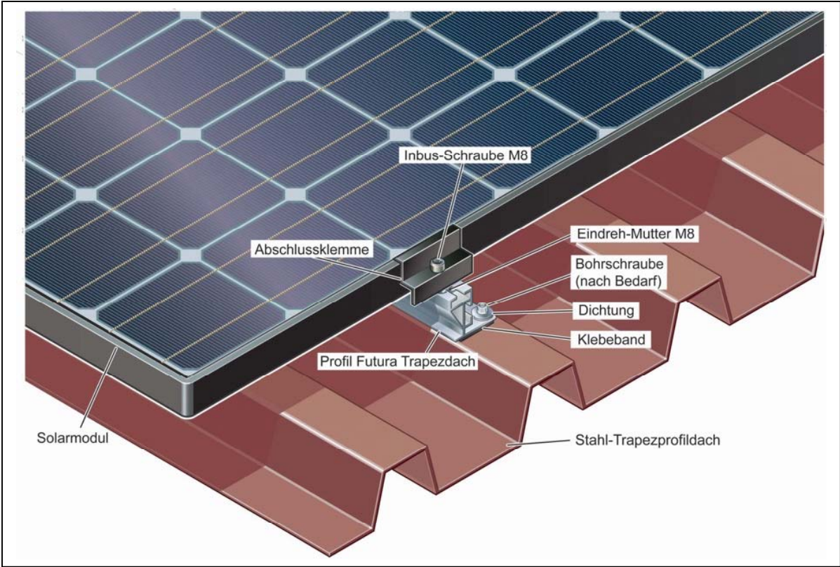
D – Trapezdach Detail Abschlussklemme - Zusammenbau
