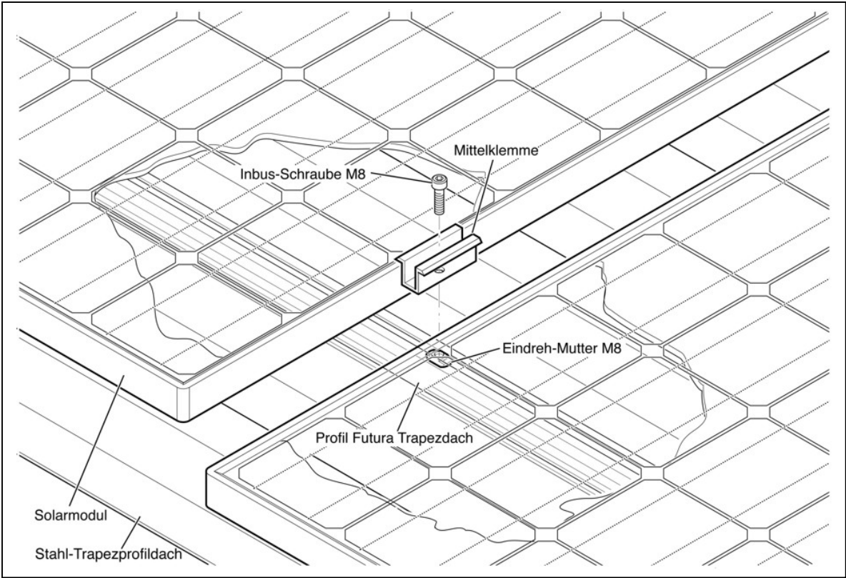
E – Trapezdach Detail Mittelklemme - Explosionsdarstellung
