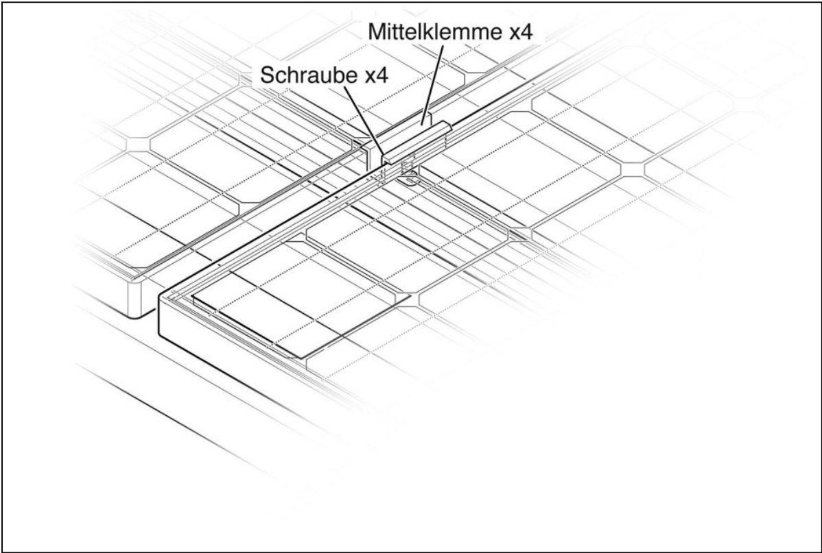
E – Trapezdach Detail Mittelklemme - Zusammenbau
