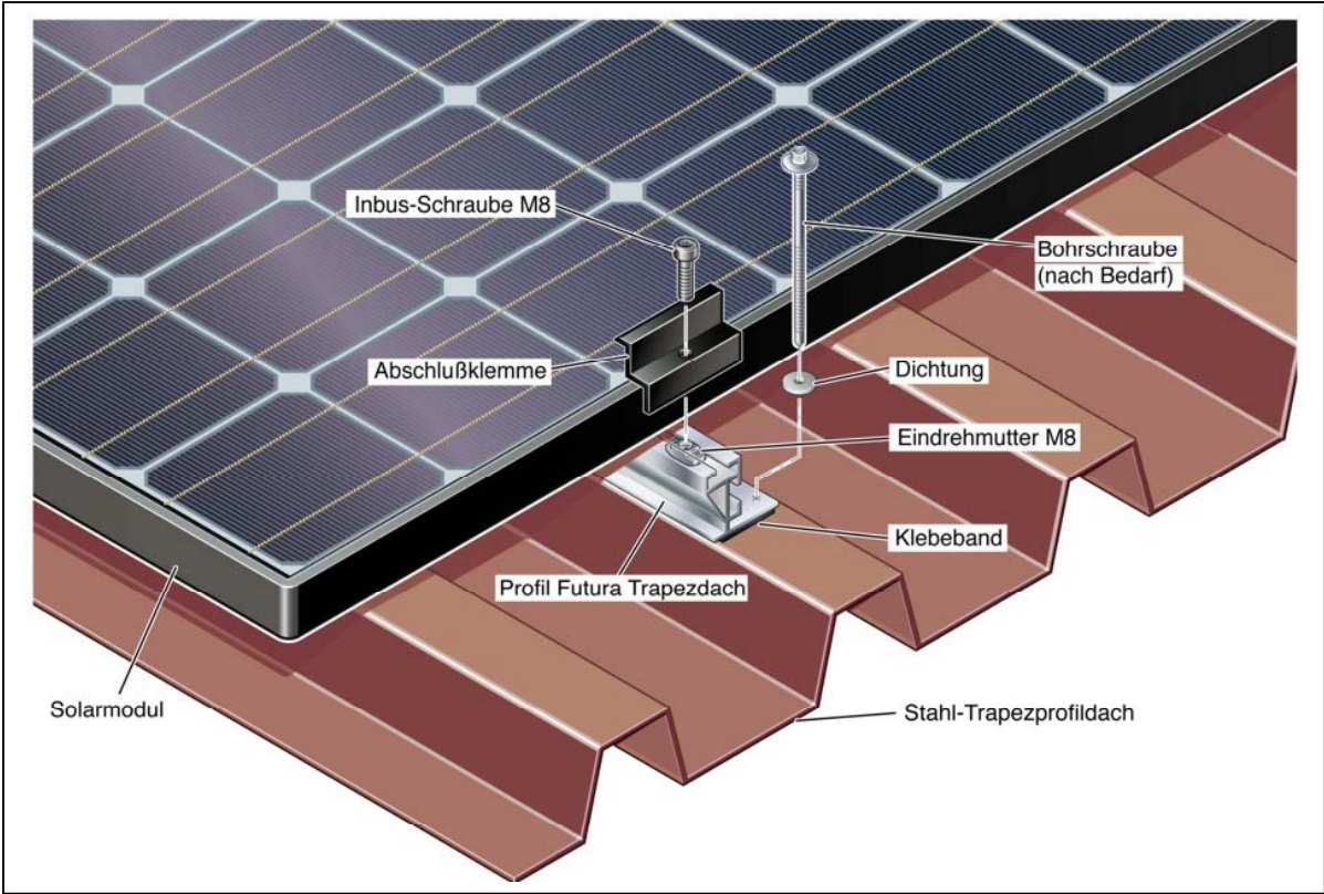
C – Trapezdach Detail Abschlussklemme - Explosionsdarstellung
