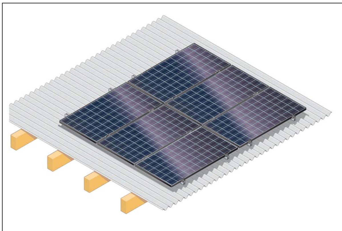
B - Module auf Welleleitndach - Zusammenbau
