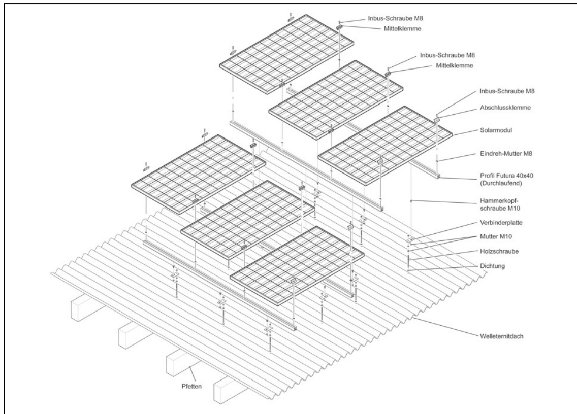
A - Modul auf Welleleitndach - Explosionsdarstellung
