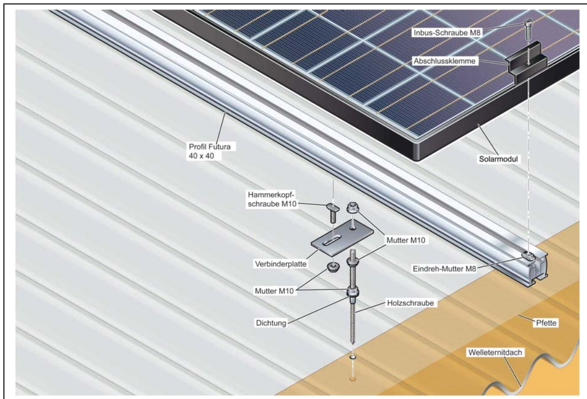
C – Wellenitndach Detail Wellenitverbindung - Explosionsdarstellung
