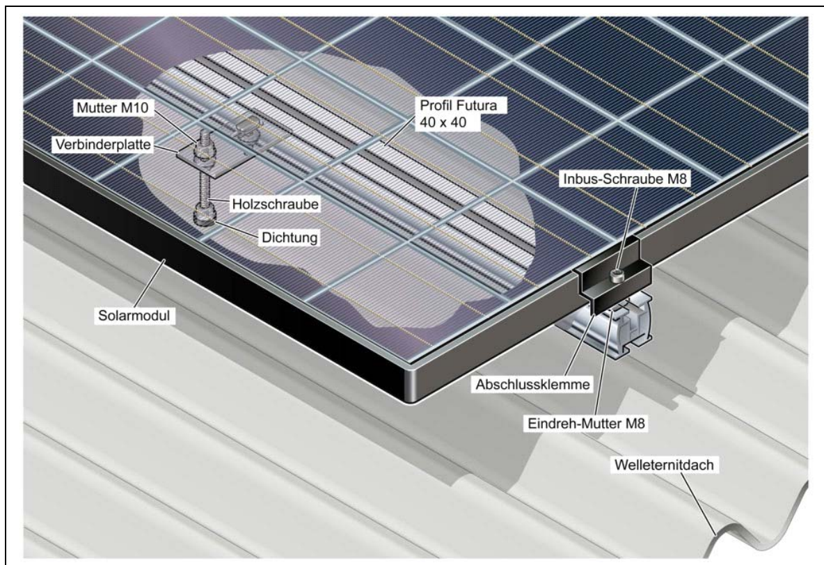
D – Wellenitndach Detail Wellenitverbindung - Zusammenbau
